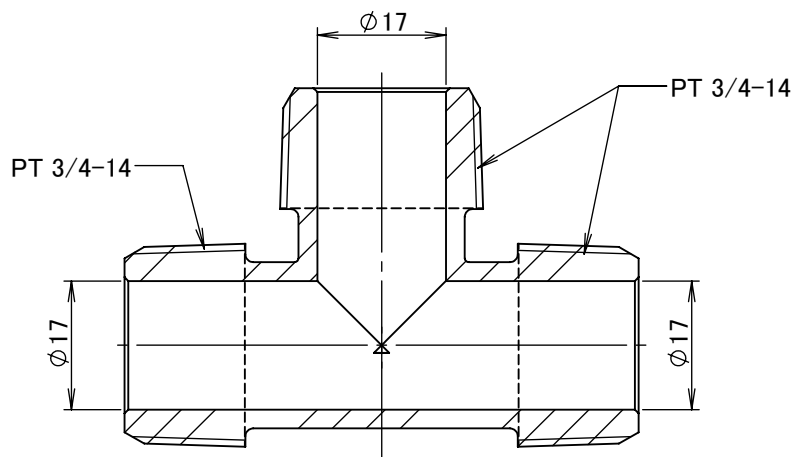
断面図 A-A
