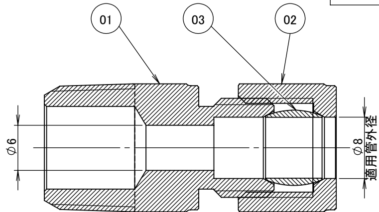
断面図 A-A
