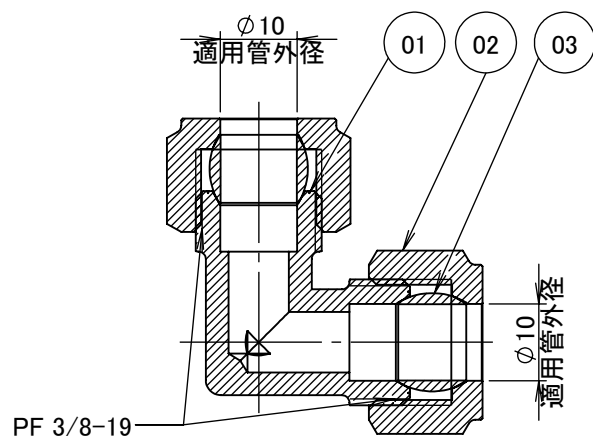
断面図 A-A
