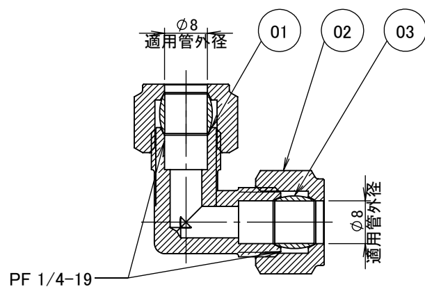
断面図 A-A
