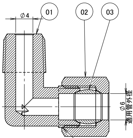
断面図 A-A
