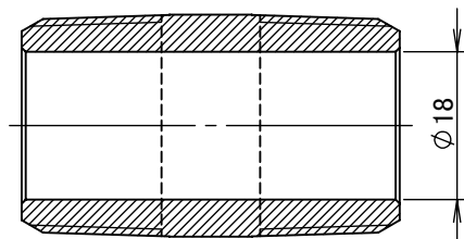
断面図 A-A
