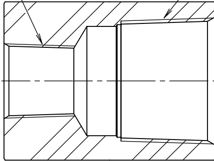
断面図 A-A
