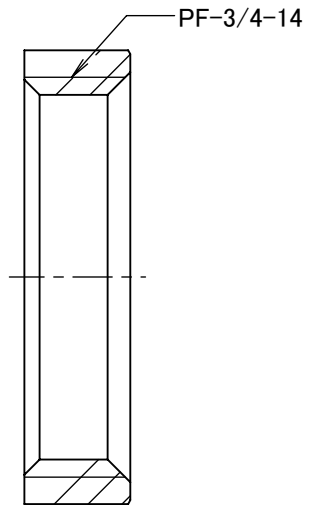
断面図 A-A
