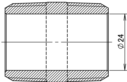
断面図 A-A
