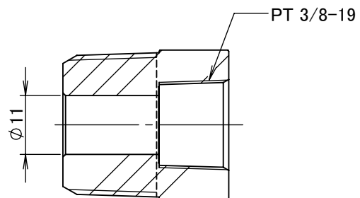
断面図 A-A
