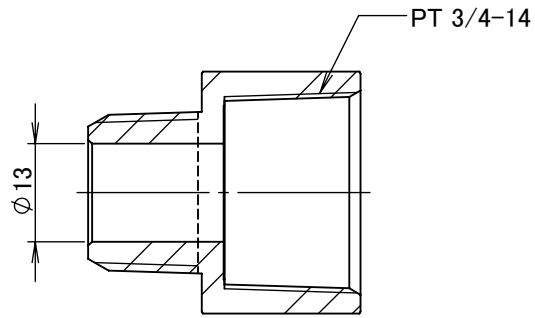
断面図 A-A
