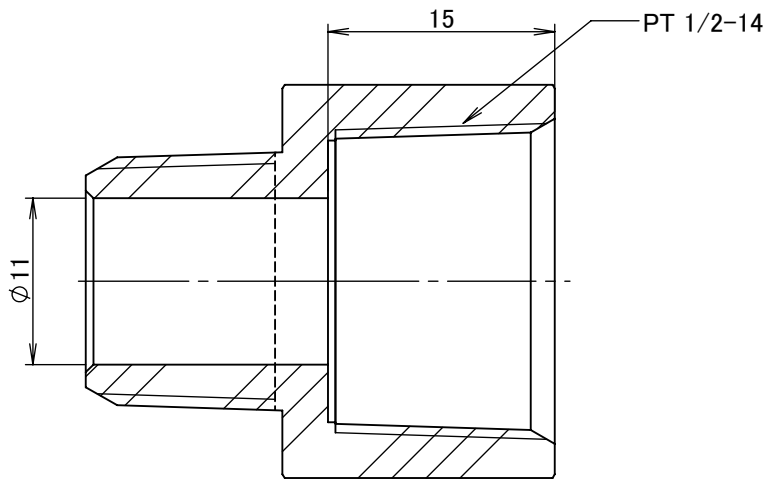
断面図 A-A
