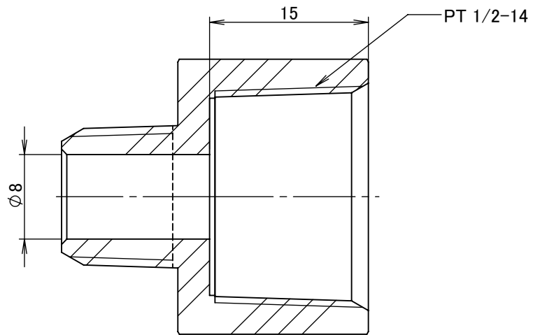
断面図 A-A
