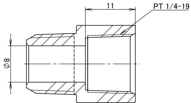
断面図 A-A
