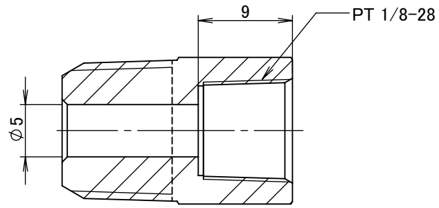
断面図 A-A
