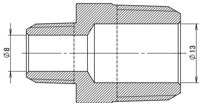
断面図 A-A
