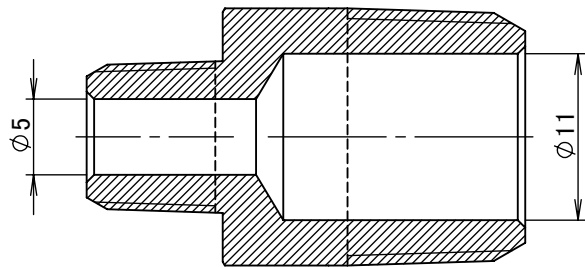
断面図 A-A
