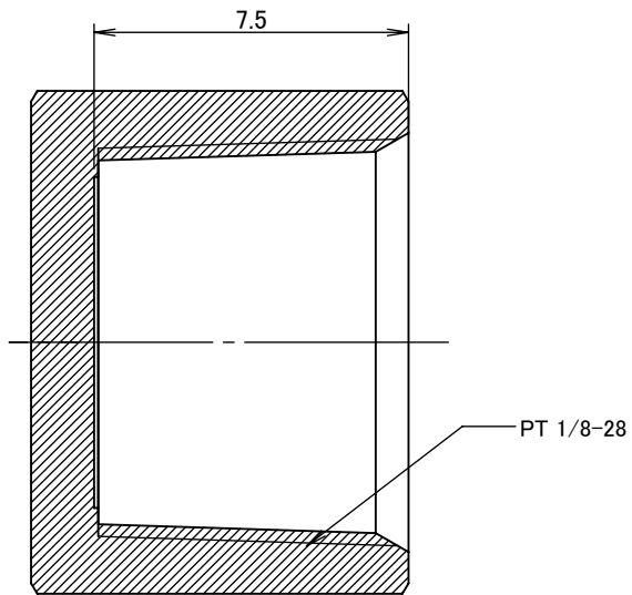
断面図 A-A
