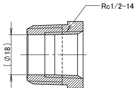
断面図 A-A
