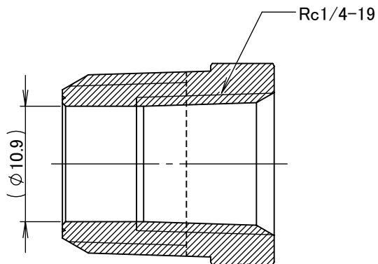
断面図 A-A
