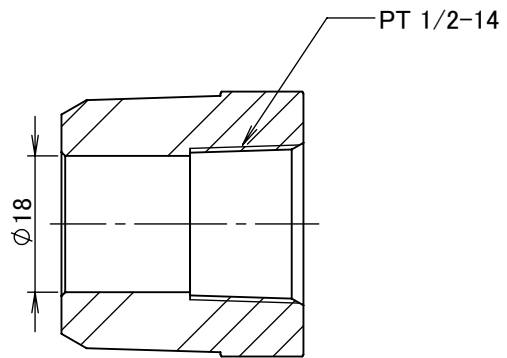
断面図 A-A
