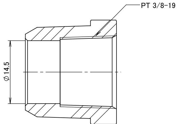
断面図 A-A
