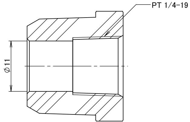
断面図 A-A
