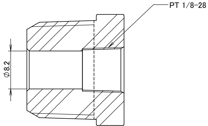
断面図 A-A
