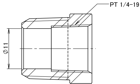
断面図 A-A
