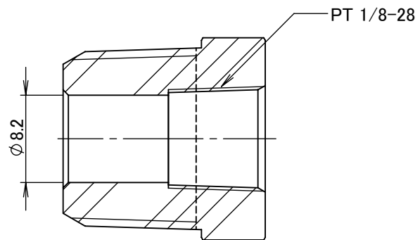
断面図 A-A
