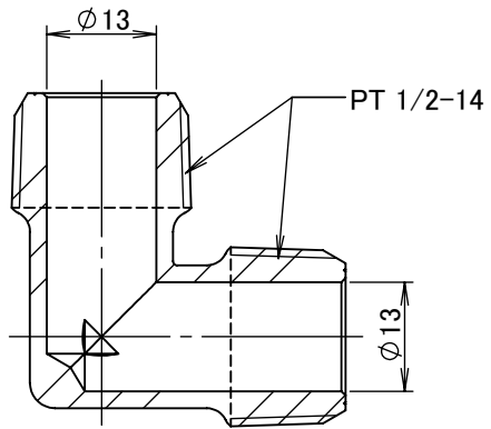
断面図 A-A
