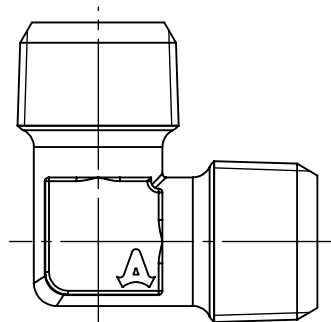
断面図 A-A
