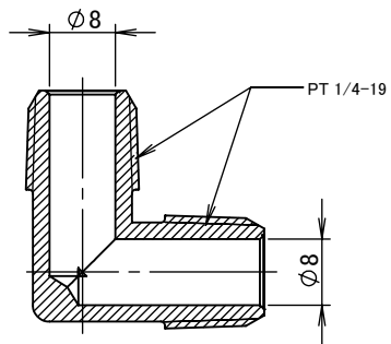
断面図 A-A
