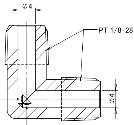
断面図 A-A
