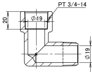
断面図 A-A
