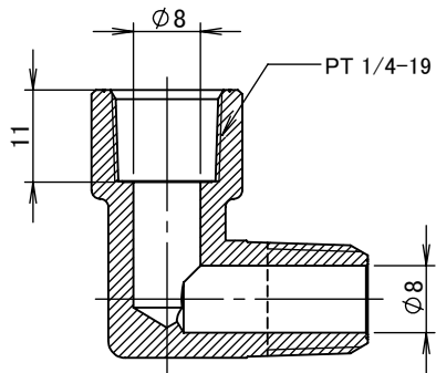
断面図 A-A
