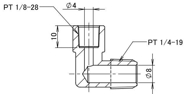
断面図 A-A
