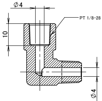
断面図 A-A
