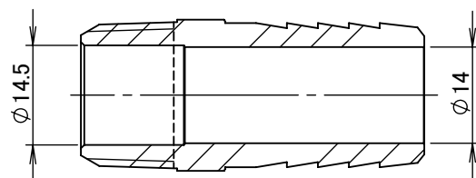
断面図 A-A
