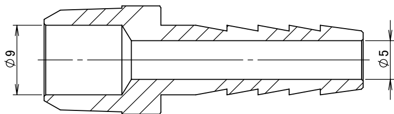
断面図 A-A
