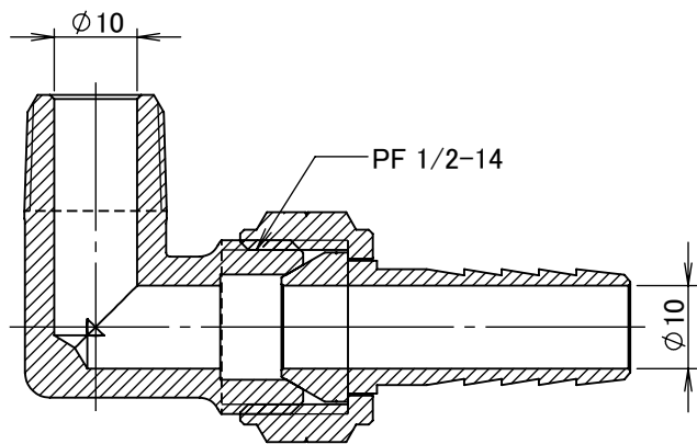
断面図 A-A
