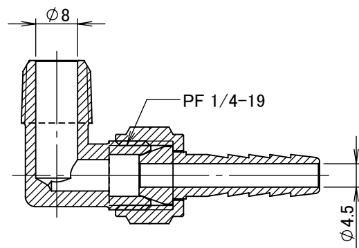
断面図 A-A
