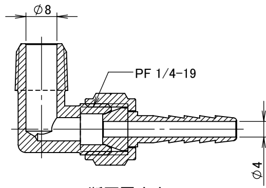
断面図 A-A
