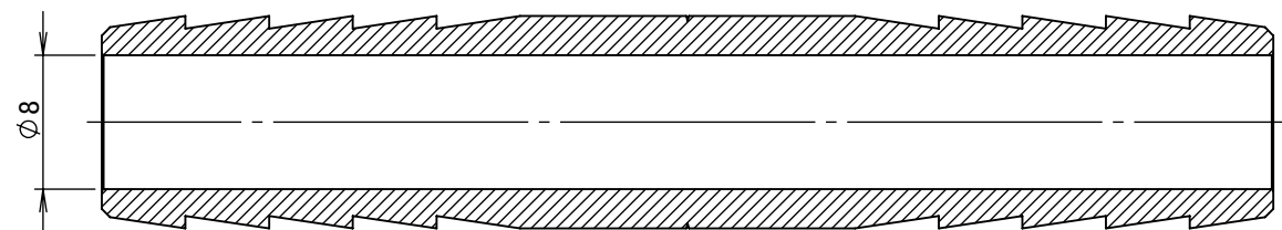
断面図 A-A
