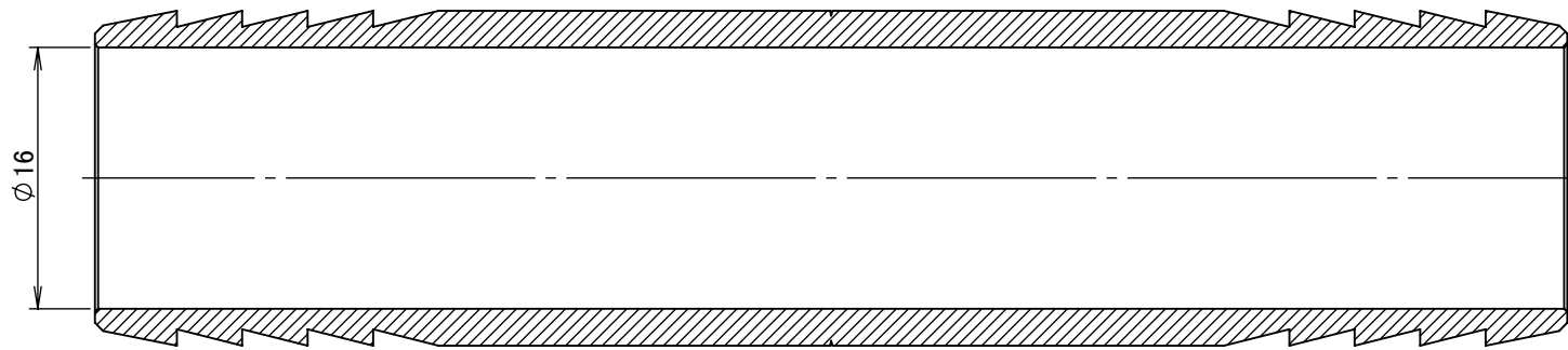
断面図 A-A
