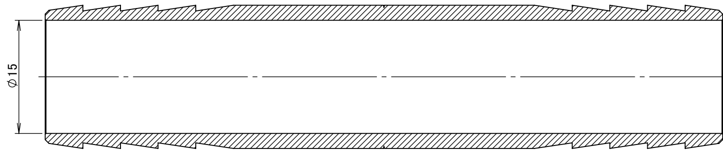
断面図 A-A
