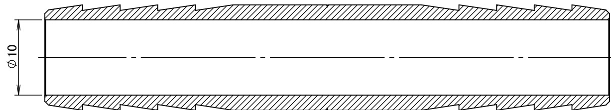
断面図 A-A
