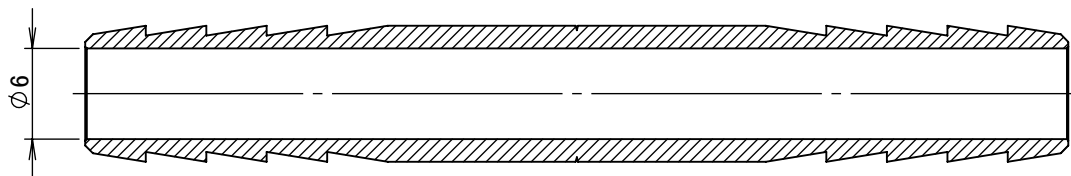
断面図 A-A
