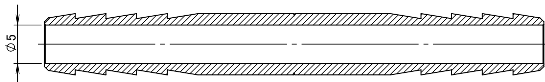
断面図 A-A
