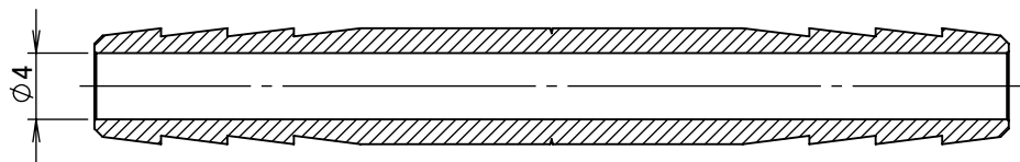
断面図 A-A
