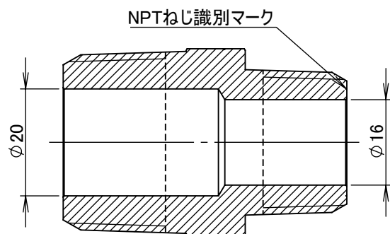
断面図 A-A
