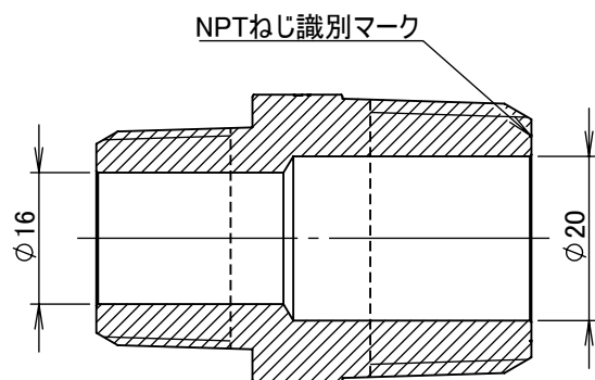
断面図 A-A
