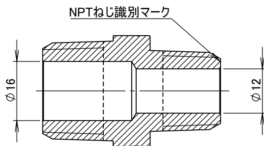
断面図 A-A
