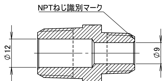
断面図 A-A
