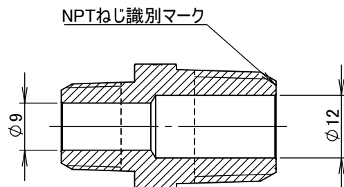
断面図 A-A
